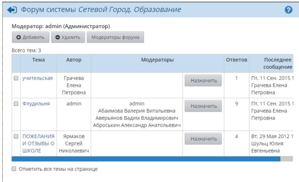
Рисунок 1 - Экран Форум
